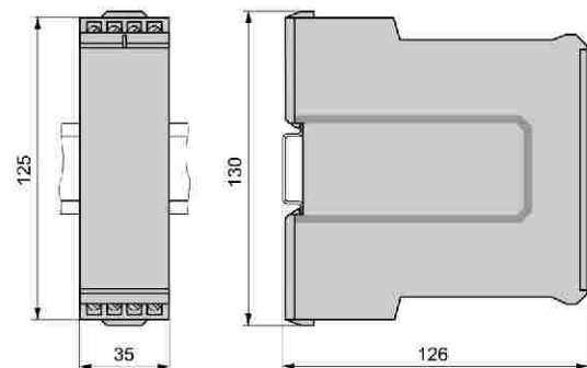
Fig. 12. Transducer clipped onto a top hat rail ( 35 \cdot 15 mm or 35 \cdot 7.5 mm) acc. to EN 50 022.
